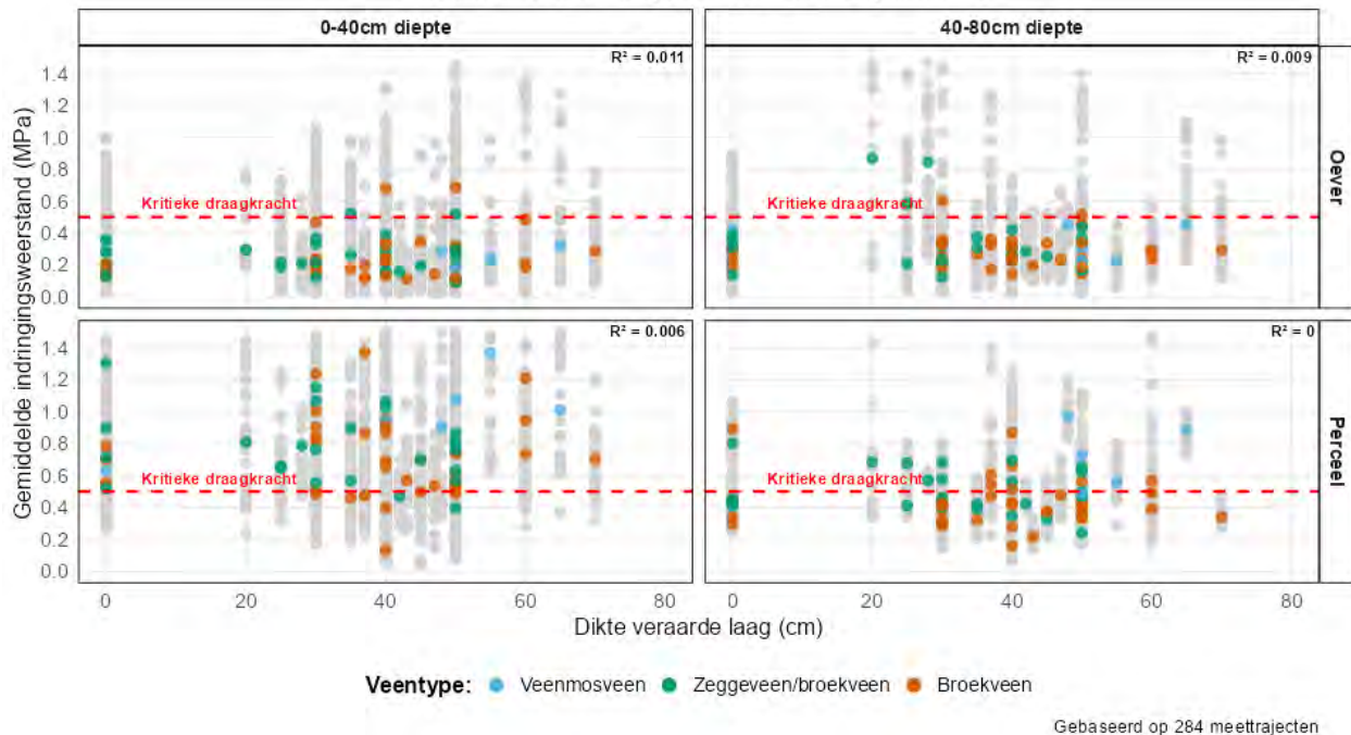
Figuur 8-4: Relatie draagkracht en drooglegging bovenste figuur en tussen draagkracht en dikte van de veraarde toplaag (onderste figuur). De grijze punten zijn de individuele metingen en de gekleurde punten zijn gebiedsgemiddelden waarbij de kleur het veentype aangeven. Links is de gemiddelde draagkracht van de bovenste 40cm en rechts van de bodemlaag 40 tot 80cm. Boven zijn de metingen in de oever en onder in het perceel.
