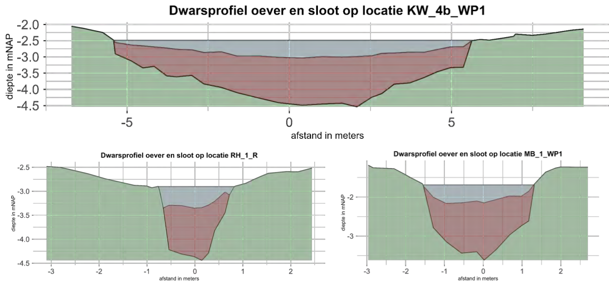
Figuur 3-14 Voorbeelden van ingemeten slootprofielen: vaste bodem (groen), slibdikte (bruin) en waterdiepte (blauw). Boven van een sloot van 10 meter breed in de Krimpenerwaard en onder twee slootprofielen van sloten van 2 meter breed.
