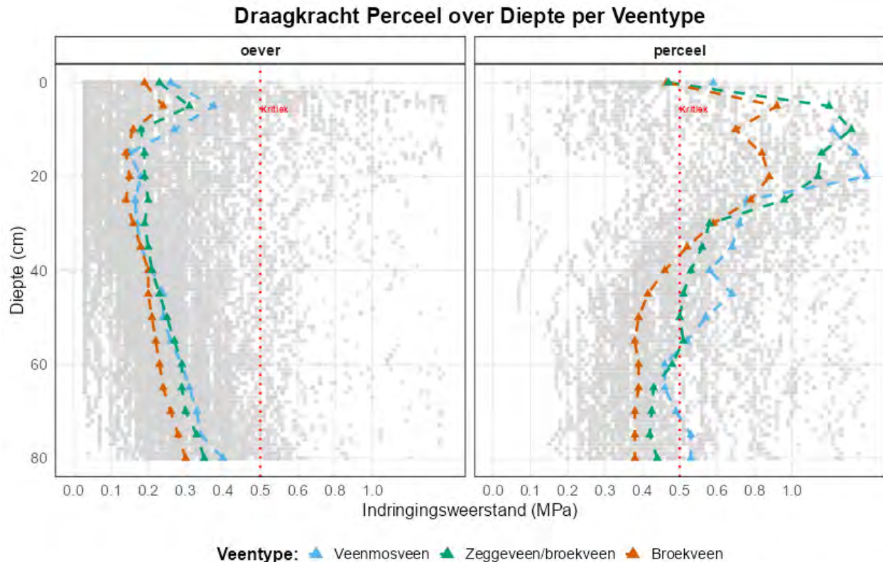
Figuur 3-22 Draagkracht gemeten op verschillende diepten ten opzichte van maaiveld. Per metpunt zijn in de oever meerdere metingen, en op het perceel één meting uitgevoerd. Mediane waarden zijn per veentype weergegeven. De lichtgrijze puntjes zijn de individuele datapunten.
