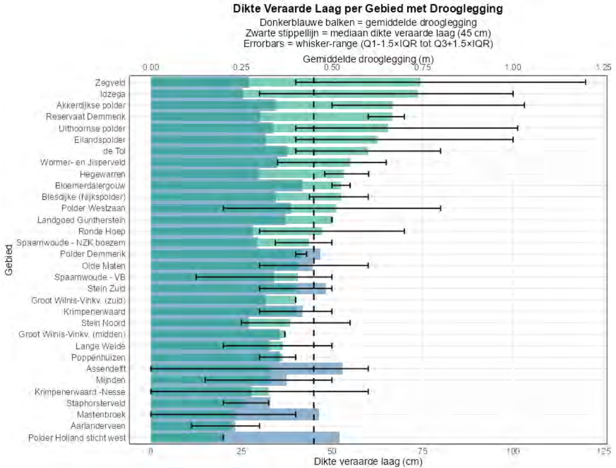
Figuur 3-20 Dikte veraarde toplaag in cm (groene balken, onderas) en de gemeten drooglegging tijdens de inventarisatie (bovenas; blauwe balken op de achtergrond). De errorbars tonen de spreiding van de data ten opzichte van de mediaan. Outliers worden niet getoont omdat de spreiding is berekend op basis van de whisker-range (Q1-1.5×IQR tot Q3+1.5×IQR), net zoals in boxplots. nee
